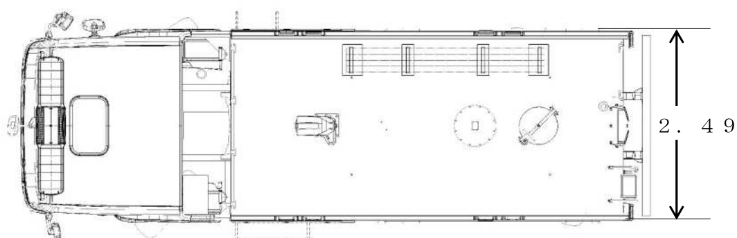
平 面 図 (単位 m)
