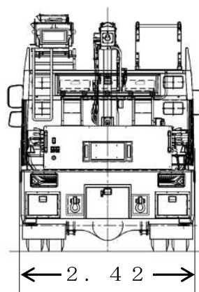
背 面 図 (単位 m)
