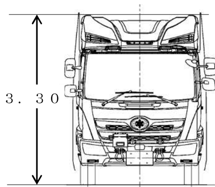
正 面 図 (単位 m)
