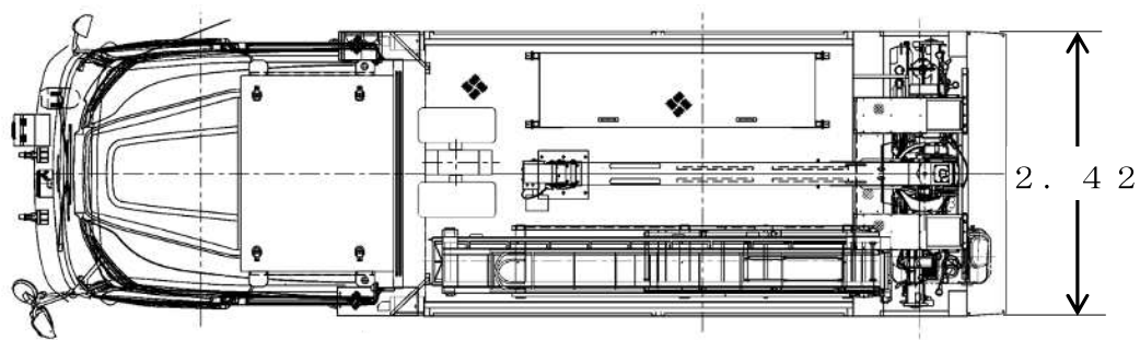
平 面 図 (単位 m)
