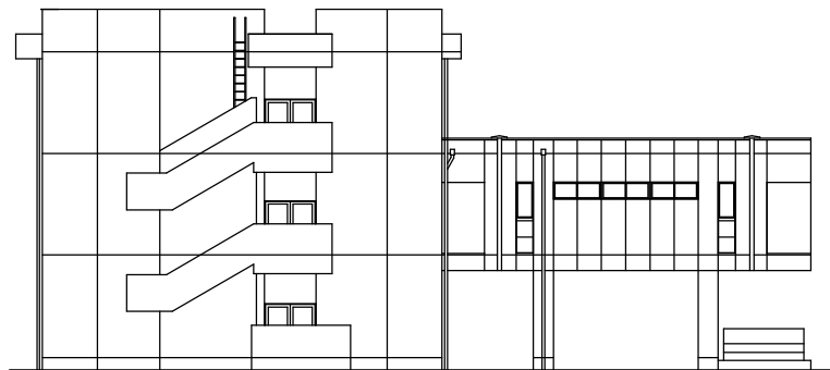
東立面图 C棟
